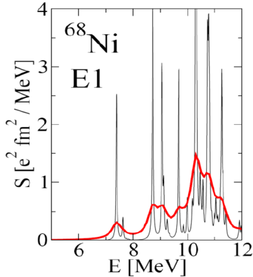
E.Litvinova et al.; PRC 79, (2009) 054312
